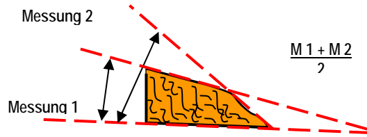
Abb. 13 Messen des Fallkerbes bei geraden und bei runden Schnitten
