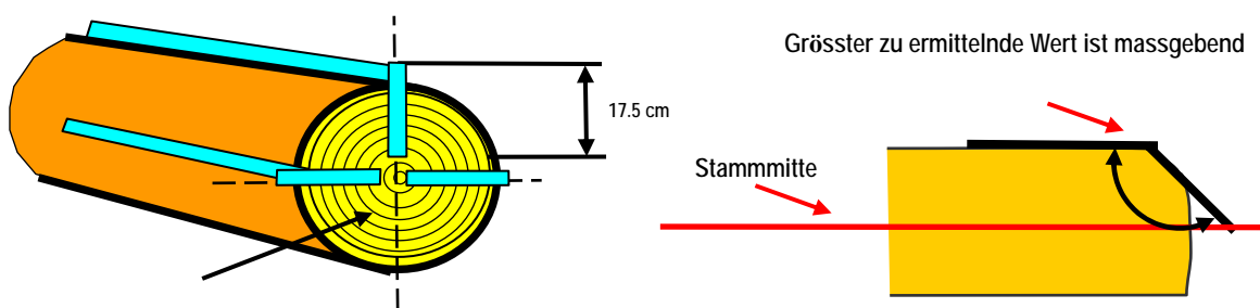
3 Messstellen beim Präzisionsschnitt
