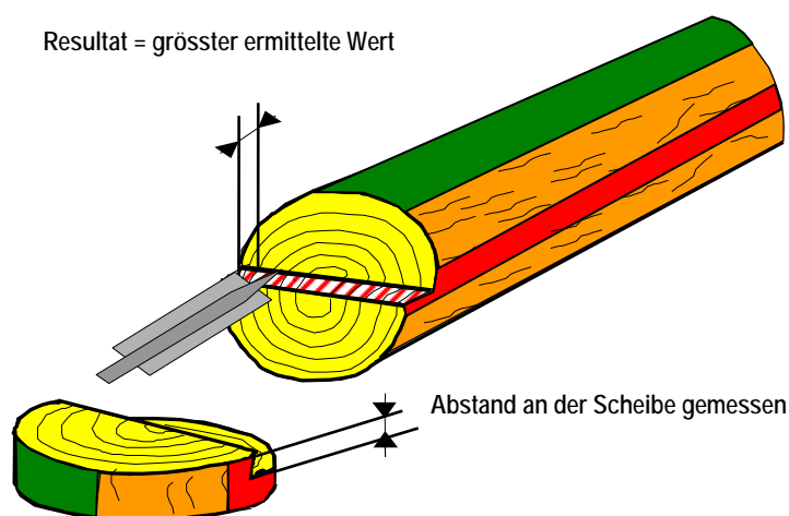
Abb. 25 Der Versatz wird am Stamm und an der Scheibe gemessen
