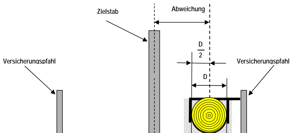
Abb. 11 Abweichung von der Fällrichtung
