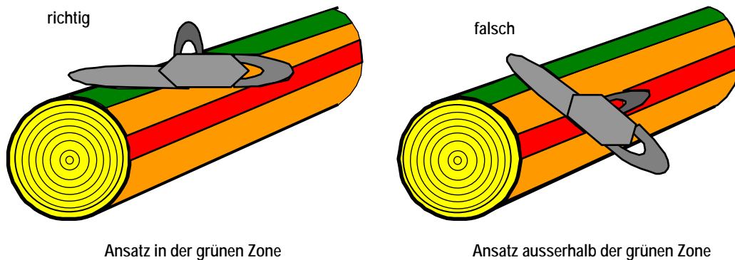
Abb. 29 Ansatz der Motorsäge beim Abwärtschnitt in der grünen Zone
