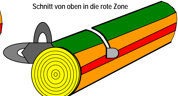
Abb. 27 Überschneiden der roten Zone von oben
