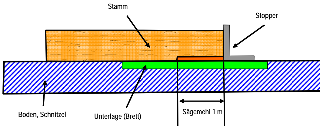
Abb. 33 Unterlage Brett und Stopper
